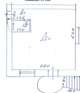
ПОЭТАЖНЫЙ ПЛАН СТРОЕНИЯ Масштаб 1:100
