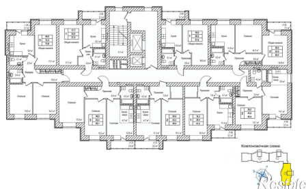
ПЛАН ТИПОВОГО ЭТАЖА пр-т ЛЕНИНГРАДСКИЙ, 53, КОРПУС 2, 3 ПОДЪЕЗД
