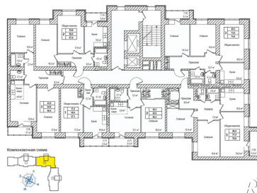
ПЛАН ТИПОВОГО ЭТАЖА пр-т ЛЕНИНГРАДСКИЙ, 53, КОРПУС 2, 2 ПОДЪЕЗД
